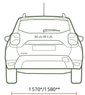
VUE ARRIÈRE
